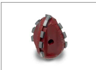
Fraise diamantée biconique- transparent - Domaine d'application: Ouverture des branchements
